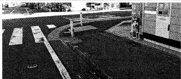
排水溝の悪臭改善 排水溝の下部に雨水等が溜まり悪臭が発生していたので、下水管の位置まで高上げしました。(古市場2丁目ファミリーマート前)
